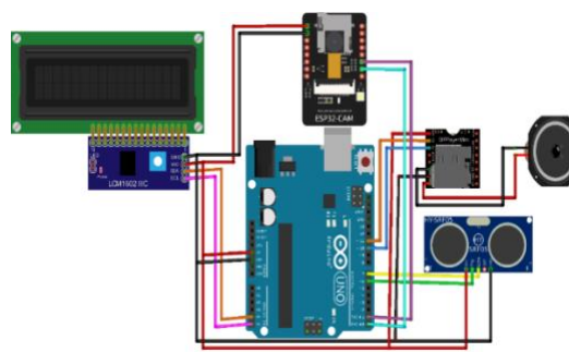
Gambar 3.1 Rangkaian Sistem
