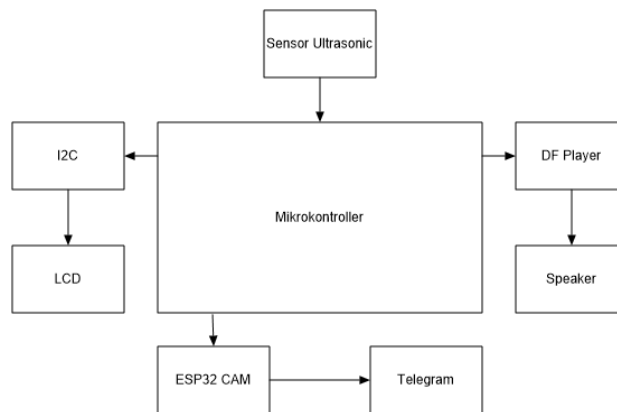
Gambar 3.2 Diagram blok desain konsep sistem.
